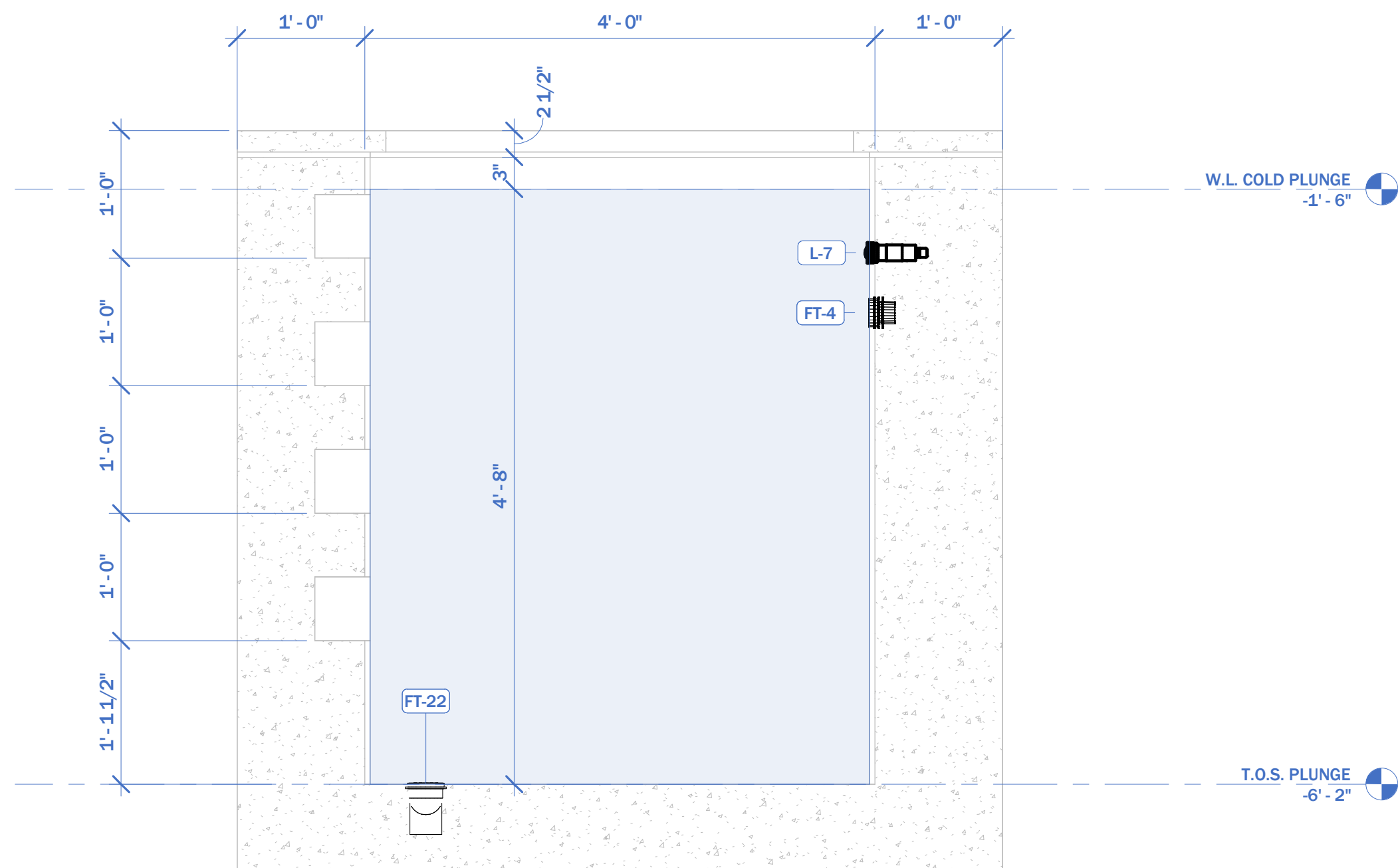
3 LONGITUDINAL COLD PLUNGE SECTION 1" = 1'-0"
